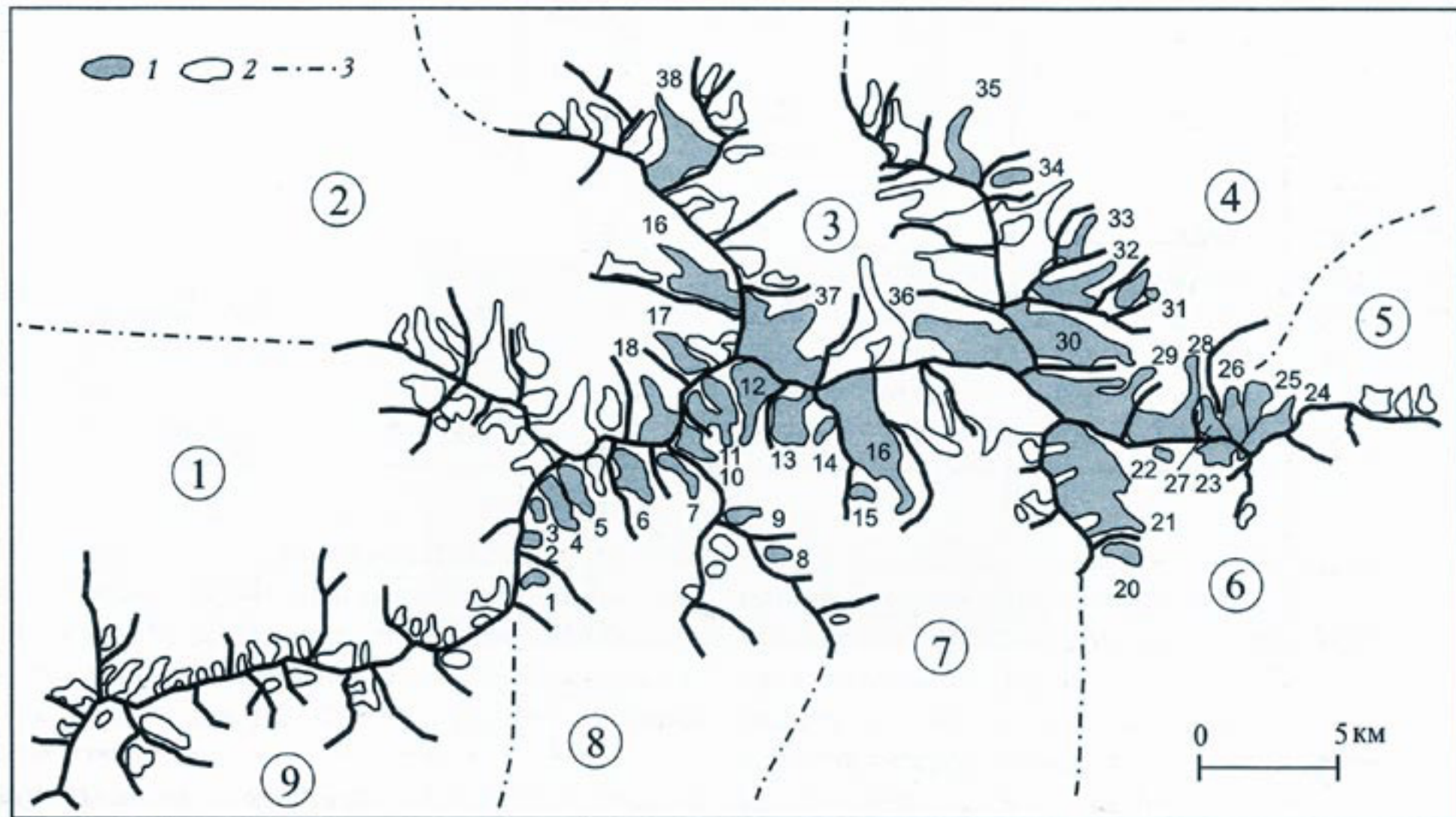
Схема района зондирования ледников Северо-Чуйского хребта. Названия бассейнов даны в табл. 1 (на рисунке они обведены кружком), а ледников — в табл. 2. Прозондированные (1) и незондированные (2) ледники; границы бассейнов (3)
