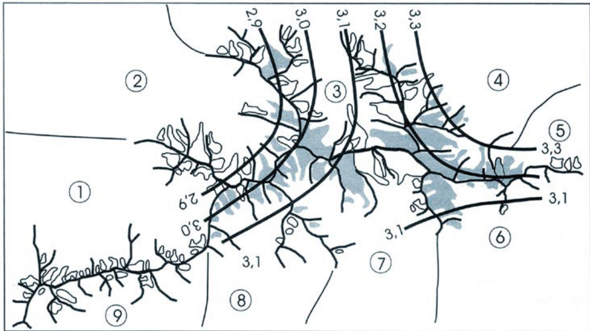
Высота зоны наибольших запасов льда Z_{vm} . (изолинии в км).
